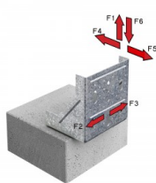
Dirección de los esfuerzos F1-F2-F3-F4-F5-F6
