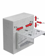
Dirección de los esfuerzos F1 hasta F6
