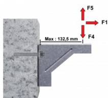
Dirección de los esfuerzos F1-F4-F5
