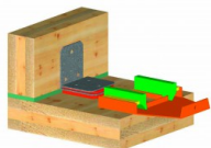
ABAI installation med MOABAI montageskabelon.
