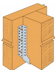
Vollausnagelung an Holz
