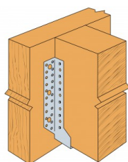
Teilausnagelung an Holz
