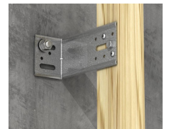
Fastgørelse af trælagte på stål
