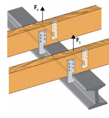
Fixation de solive avec 2 ancrages AI
