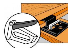
Fastgørelse af CLIP med hæfteklammer
