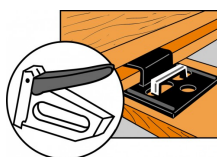
Fastgørelse af CLIP med hæfteklammer
