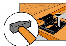
Fastgørelse af CLIP med søm
