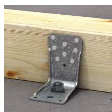
Fixation poutre sur dalle béton
