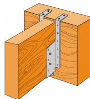
Fixation d'un sabot à bretelle avec N3.75
