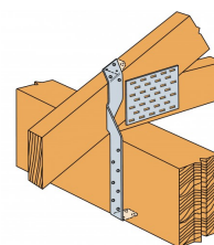
Fixation de ferme sur sablère par feuillards torsadés MTS
