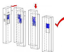
Etapes d'installation
