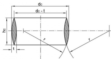
Spécification anneaux
