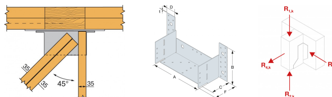
ETC485R Assemblages 2 éléments 1 arêtier double - 1 empannon
