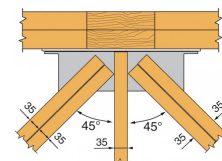
ETC835 Assemblages 3 éléments 2 arêtiers simples - 1 empannon
