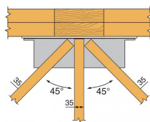
ETC835 Assemblages 3 éléments 2 arêtiers simples - 1 empannon
