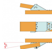
S1030 à 10° avec vis CSA ou pointes CNA
