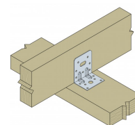
Connexion bois sur bois
