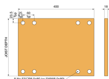
Dimension des blocs de renforts bois
