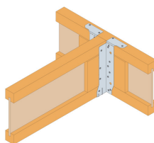
Fixation par les brides supérieures sur un support poutre en I avec renfort
