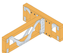
Fixation par les brides supérieures sur une poutre métallique ajourée avec renfort bois
