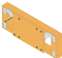
Dimension des blocs de renforts bois
