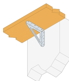
Fijación de ménsulas
