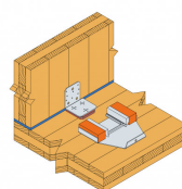
ABAI installation med MOABAI montageskabelon.
