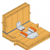
ABAI installation med MOABAI montageskabelon.
