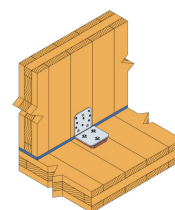
ABAI installation med SDS skruer
