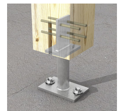
Fixation du PISB160G-K sur support rigide
