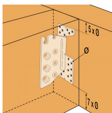
Anschluss an HT
