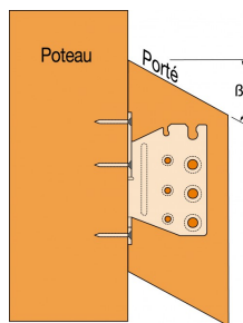
Anschluss mit Neigung an Stütze
