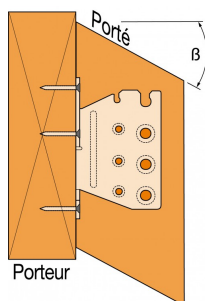
Anschluss mit Neigung an HT
