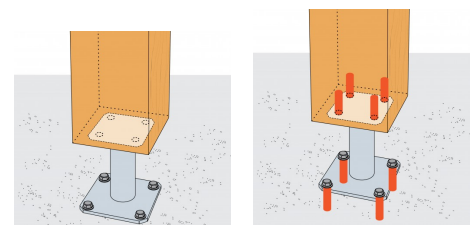
Verwendete Befestigungen für Stützenfuß Typ PPA
