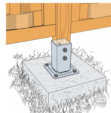
Fixation de clôtures sur support rigide
