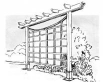
Befestigung von Pergolen auf Betonfundament
