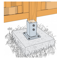
Fixation de clôtures sur support rigide
