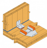
Montage de l'équerre à l'aide du gabarit
