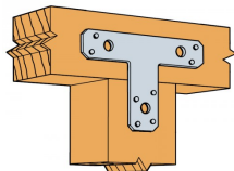
Fixation en T avec 66T
