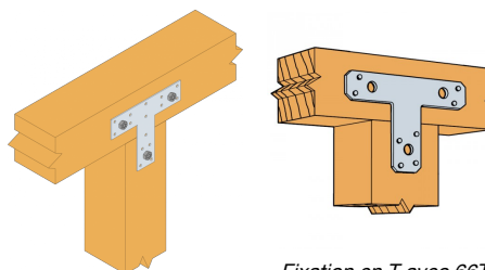
Fixation en T avec 66T
