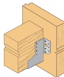
Clouage partiel sur bois.
