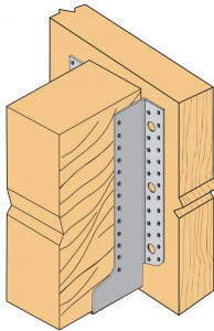
Clouage total sur bois.
