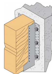
Fixation sur support rigide.
