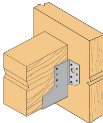
Clouage partiel sur bois.
