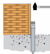
Fixation de palissades à enfoncer dans le sol
