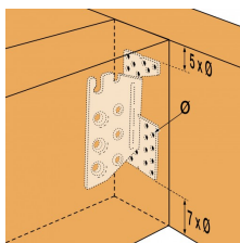
Rechte verbinding op balk
