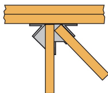
1 arêtier + 1 empannon
