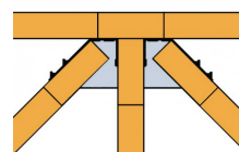
ETC392 - Verbindingen 2 enkele hoekkepers + 1 karbeel
