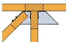
ETC 392 - Verbinding 1 karbeel + 1 linkse hoekkeper
