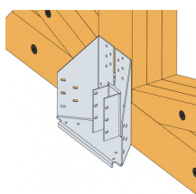
ETC 392 - Verbinding 1 karbeel + 1 rechtse hoekkeper
