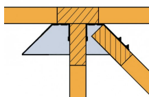
ETC 392 - Verbinding 1 karbeel + 1 rechtse hoekkeper
