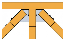
ETC392 - Verbindingen 2 enkele hoekkepers + 1 karbeel
