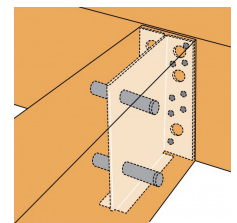
Dwarsbalkverbinding op balk
