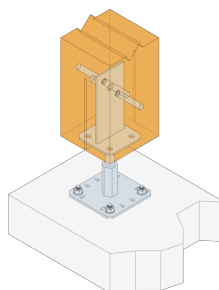
Bevestiging 2 pennen
