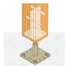
Bevestiging 2 pennen
