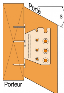
Schuine verbinding op balk
