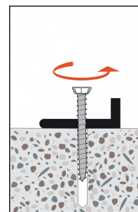
Monter la vis au travers de la pièce à fixer
