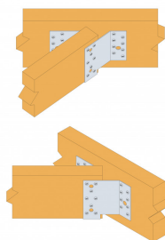
Fixation d'une poutre à 45°
