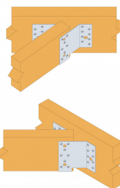
Fixation d'une poutre à 45°
