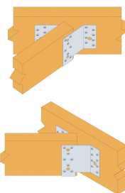
Fixation d'une poutre à 45°
