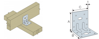
Connexion bois sur bois
