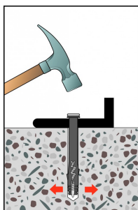
Enfoncer au marteau
