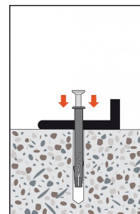
Monter la cheville au travers de la pièce à fixer
