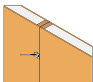
Mise en oeuvre entre panneaux bois: insérer les 2 pointes torsadées
